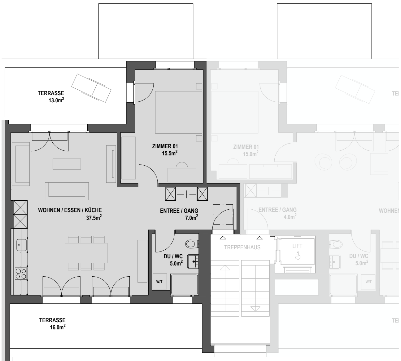
Grundriss Mst 1:100
