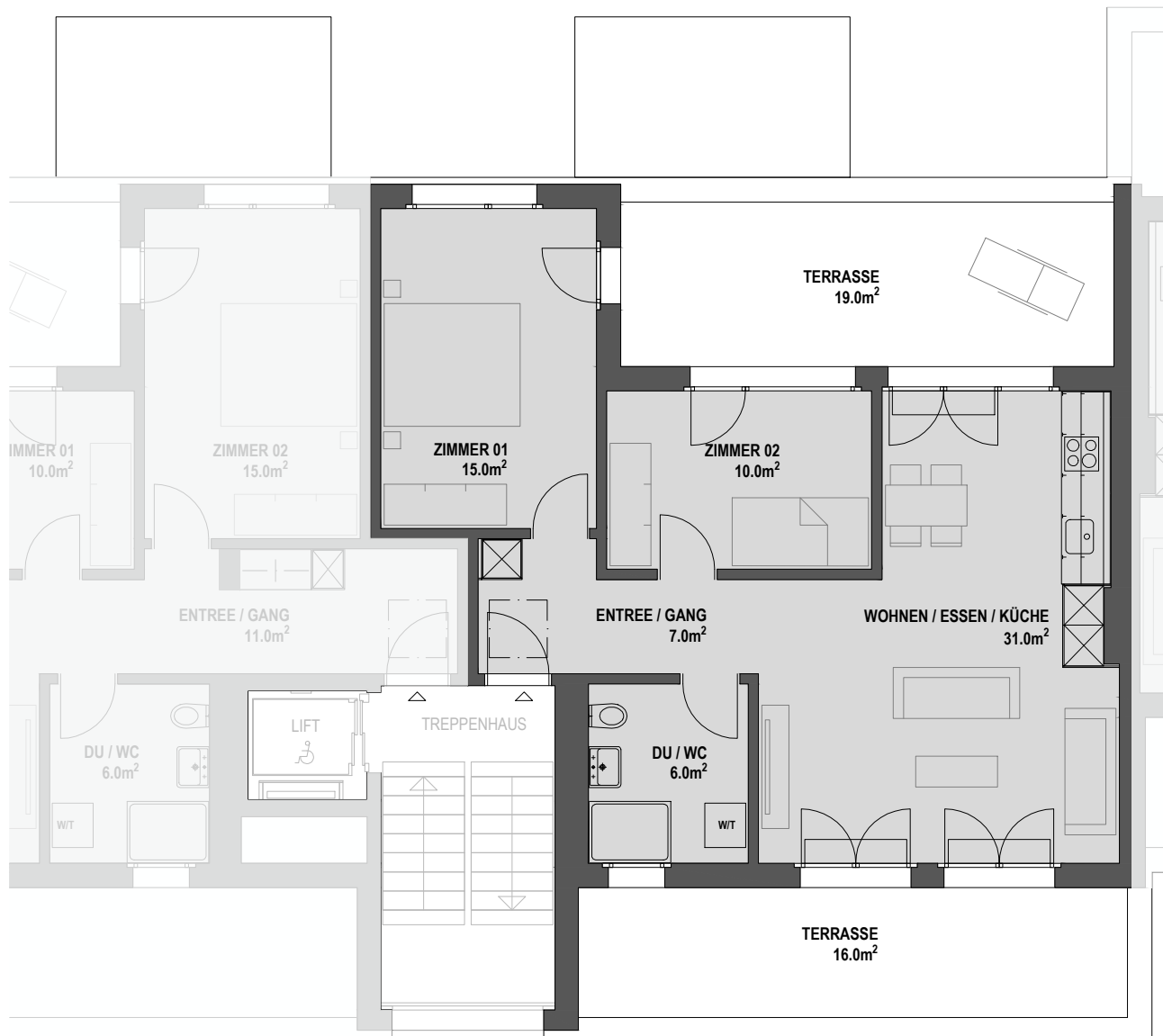
Grundriss Mst 1:100
